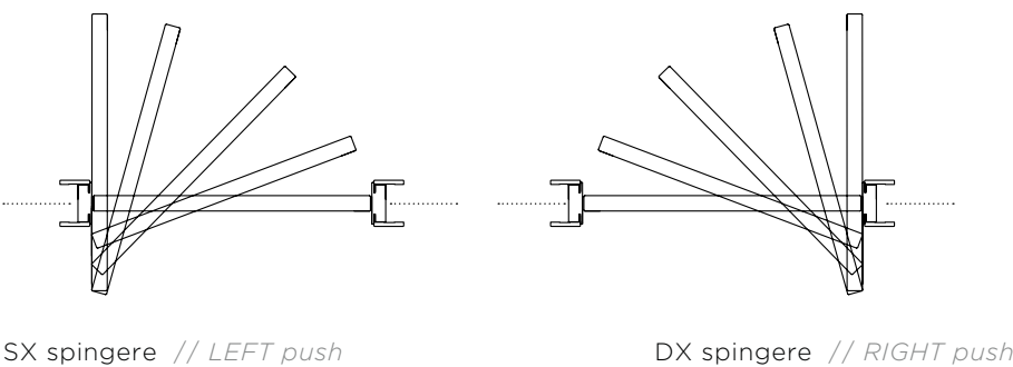
RTR — porta battente rototraslante // rotating-hinged door
