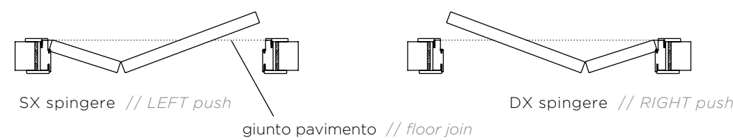
PAS — porta pieghevole pacchetto 1/3 + 2/3 // folding door 1/3 + 2/3
