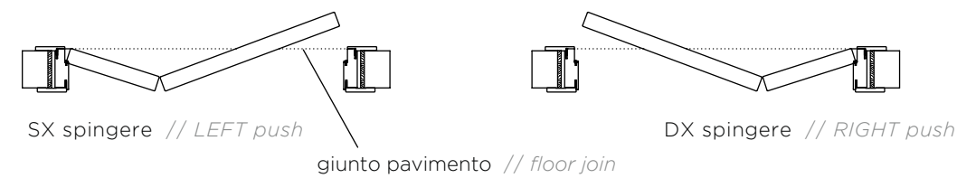
PAS — porta pieghevole pacchetto 1/3 + 2/3 // folding door 1/3 + 2/3
